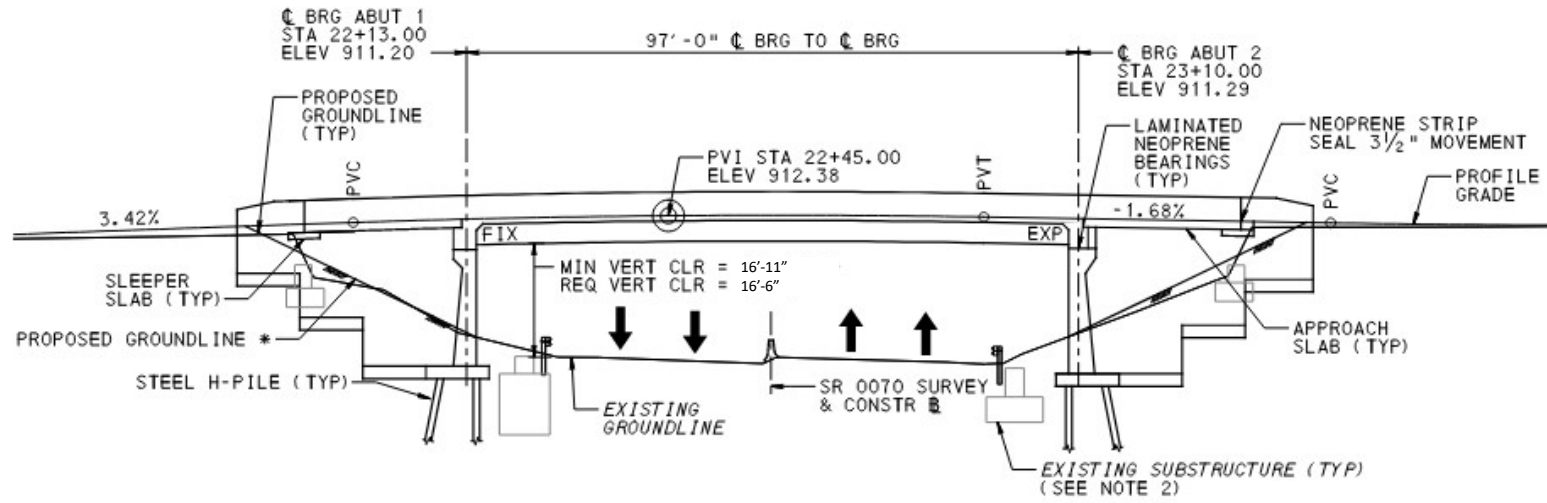
ELEVATION
